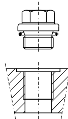
Plug met rand en elastische borgring
