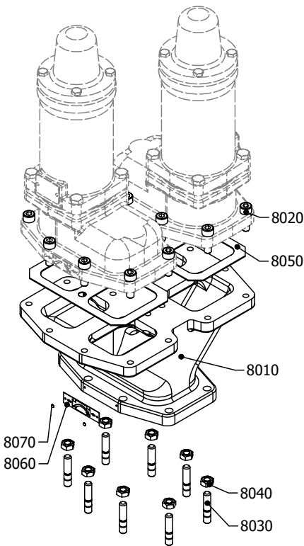
Dubbele veiligheidsklep – verticaal
