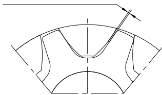
Speling tussen tanden van de tandwielen
