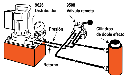
Cilindros de doble efecto controlados por una válvula montada de forma remota.
