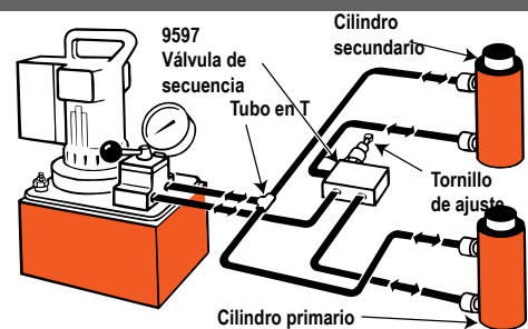
Cilindros de doble efecto con válvula de secuencia que controla los circuitos de los cilindros primario y secundario.
