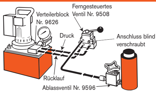
3 System mit Einfachwirkendem Zylinder, Betätigung über ein ferngesteuertes Ventil.
