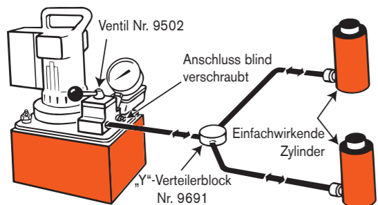
1 System mit Einfachwirkendem Zylinder(n), Steuerung über ein auf der Pumpe montiertes Ventil.
