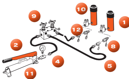
System mit Handpumpe, Manometer, Schläuchen, Absperrventilen, Ablassventilen und mehreren einfachwirkenden Zylindern.
