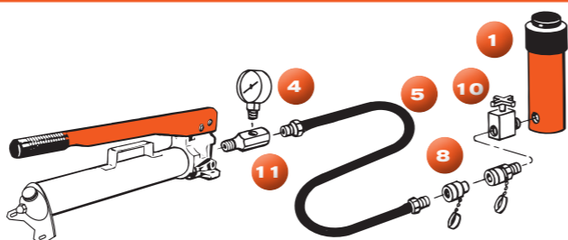
System mit Handpumpe, Manometer, Schlauch und einfachwirkendem Zylinder.
