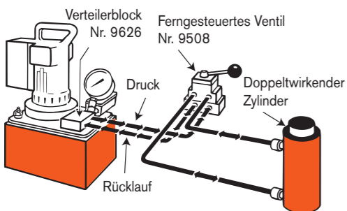
4 Doppeltwirkende Zylinder, Steuerung über ferngesteuertes Ventil.
