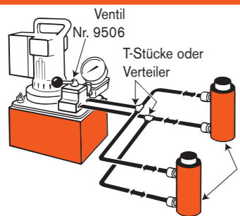
2 System mit Doppeltwirkendem Zylinder, Steuerung über ein auf der Pumpe montiertes Ventil.
