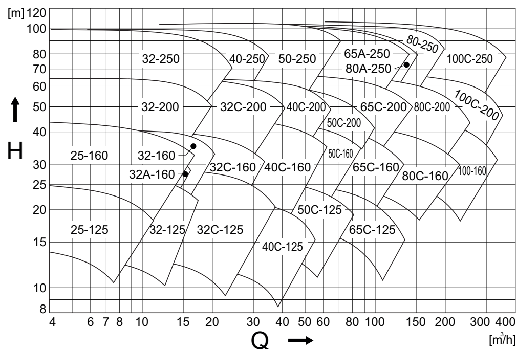
Рисунок 20: Обзор рабочих параметров при 3000 мин -1 .
