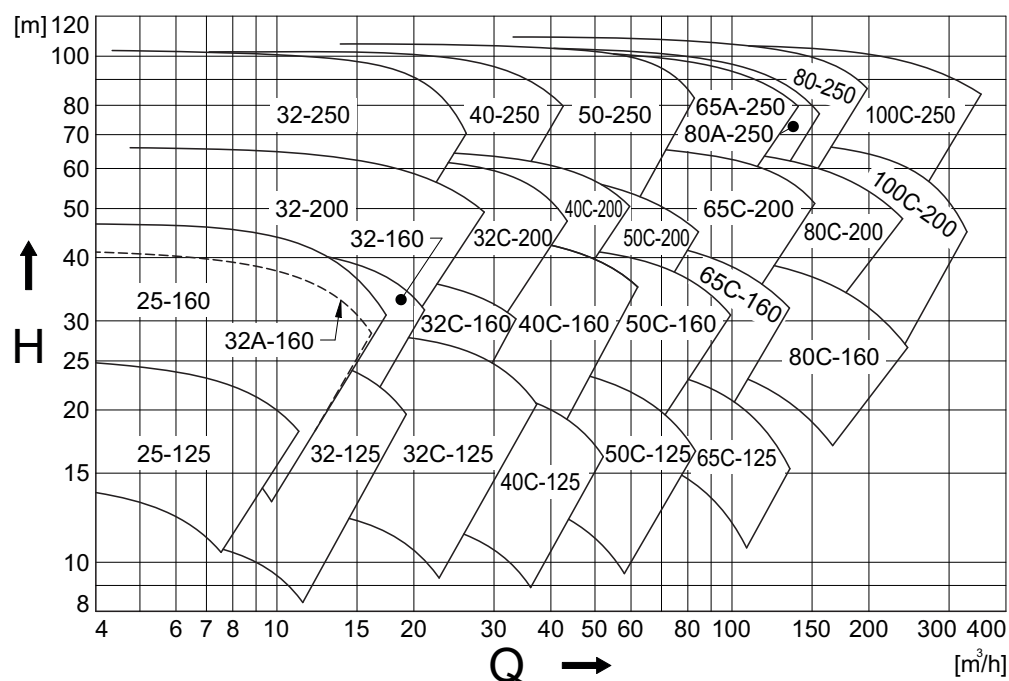
Рисунок 26: Обзор рабочих параметров при 3000 мин -1 .
