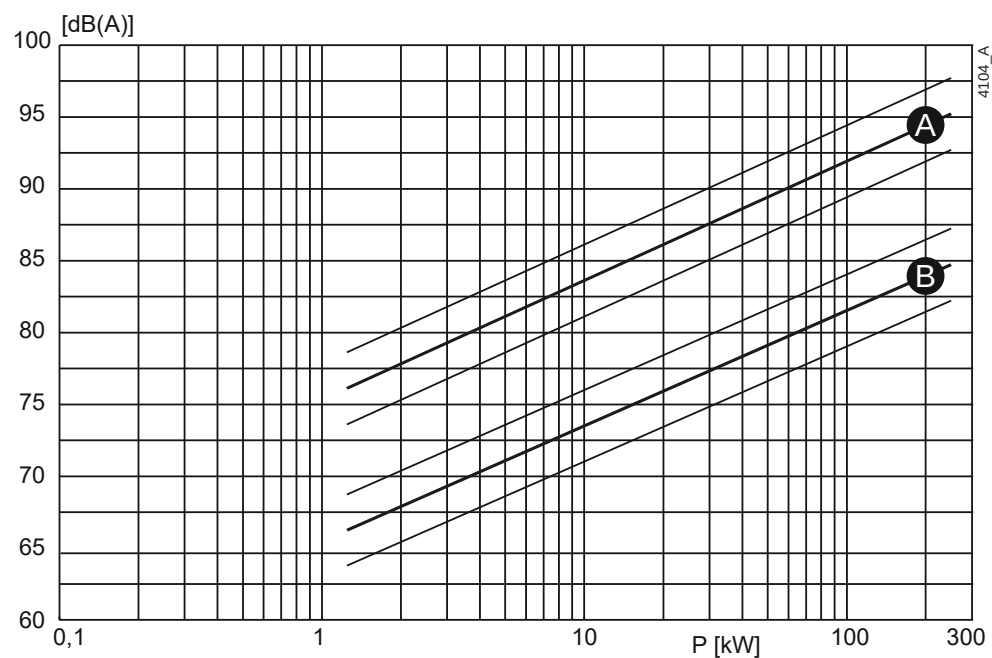
Рисунок 32: Зависимость уровня шума от мощности насоса [кВт] при 2900 \text{ мин}^{-1}
