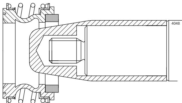
Рисунок 10: Специальная монтажная втулка.
