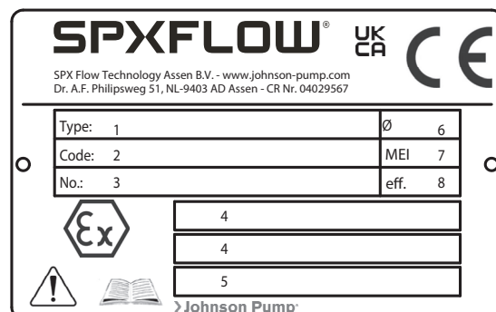
Рисунок 5: Сертифицированная ATEX заводская табличка
