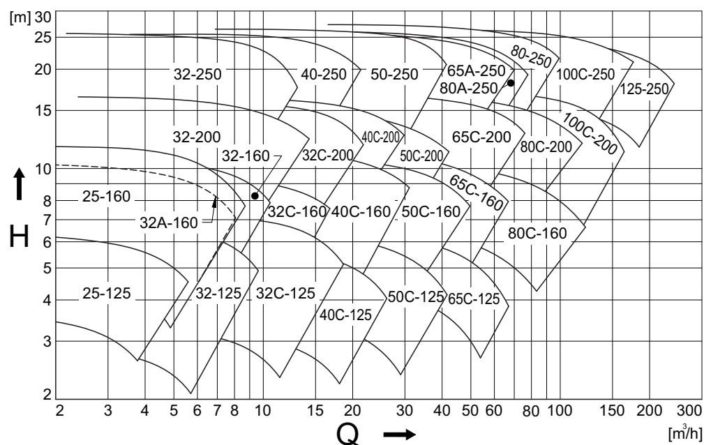
Рисунок 27: Обзор рабочих параметров при 1500 мин -1 .
