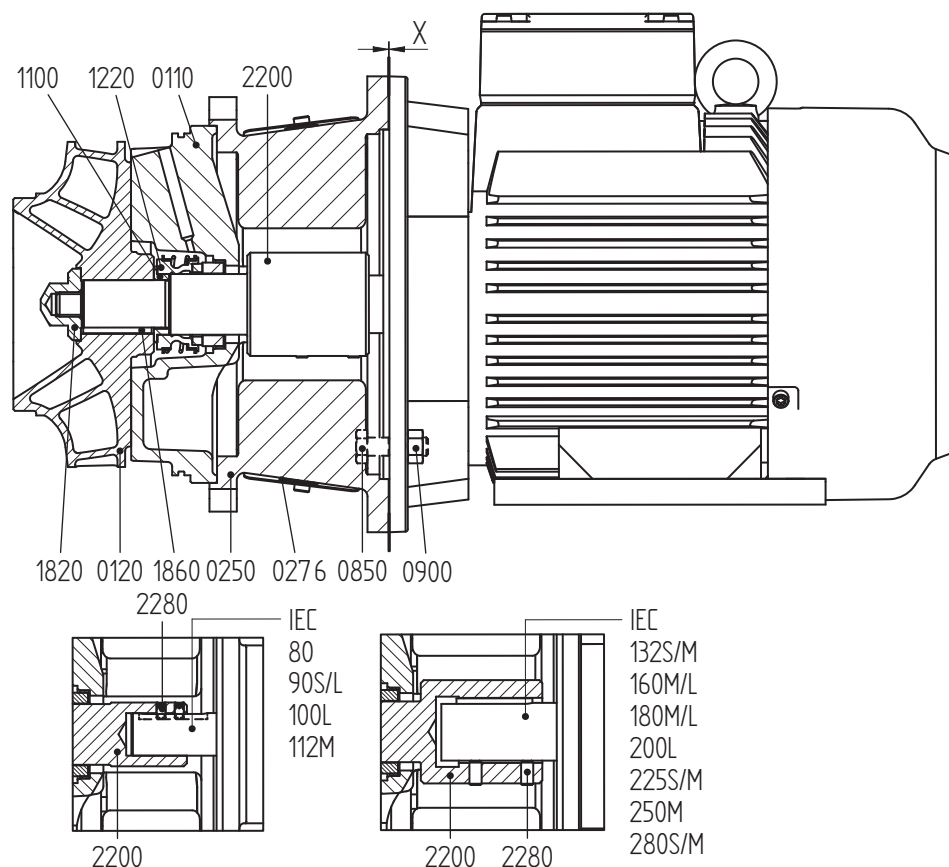
Рисунок 14: Сборка втулочного вала
