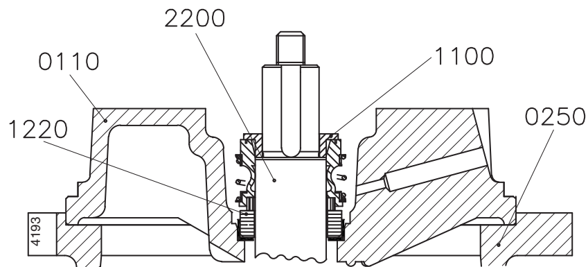
Рисунок 11: Механическое уплотнение M1.
