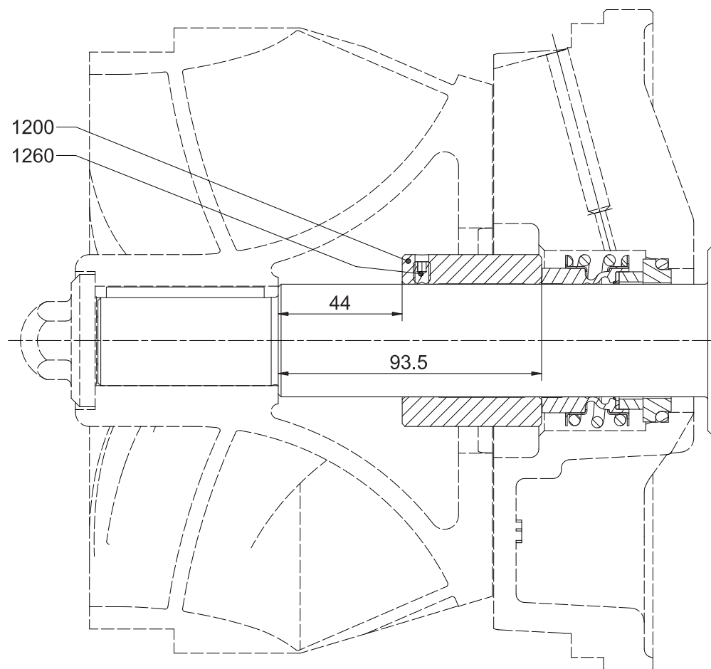
Рисунок 19: Втулка вала для 200-160.
