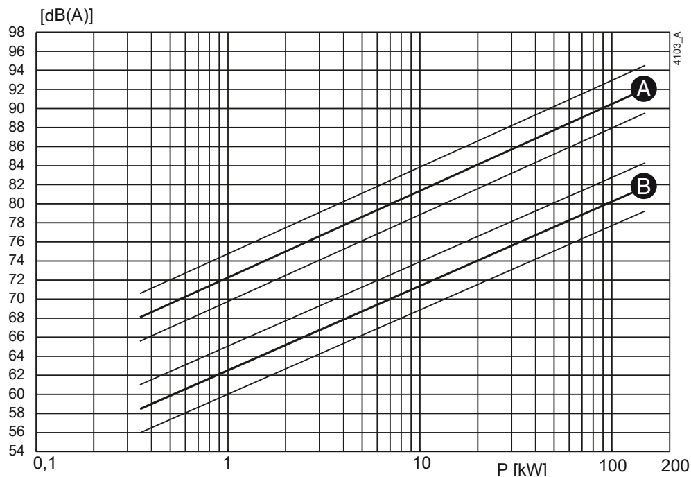
Рисунок 31: Зависимость уровня шума от мощности насоса [кВт] при 1450 \text{ мин}^{-1}
