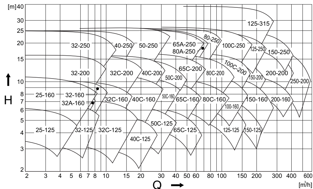
Рисунок 21: Обзор рабочих параметров при 1500 мин -1 .
