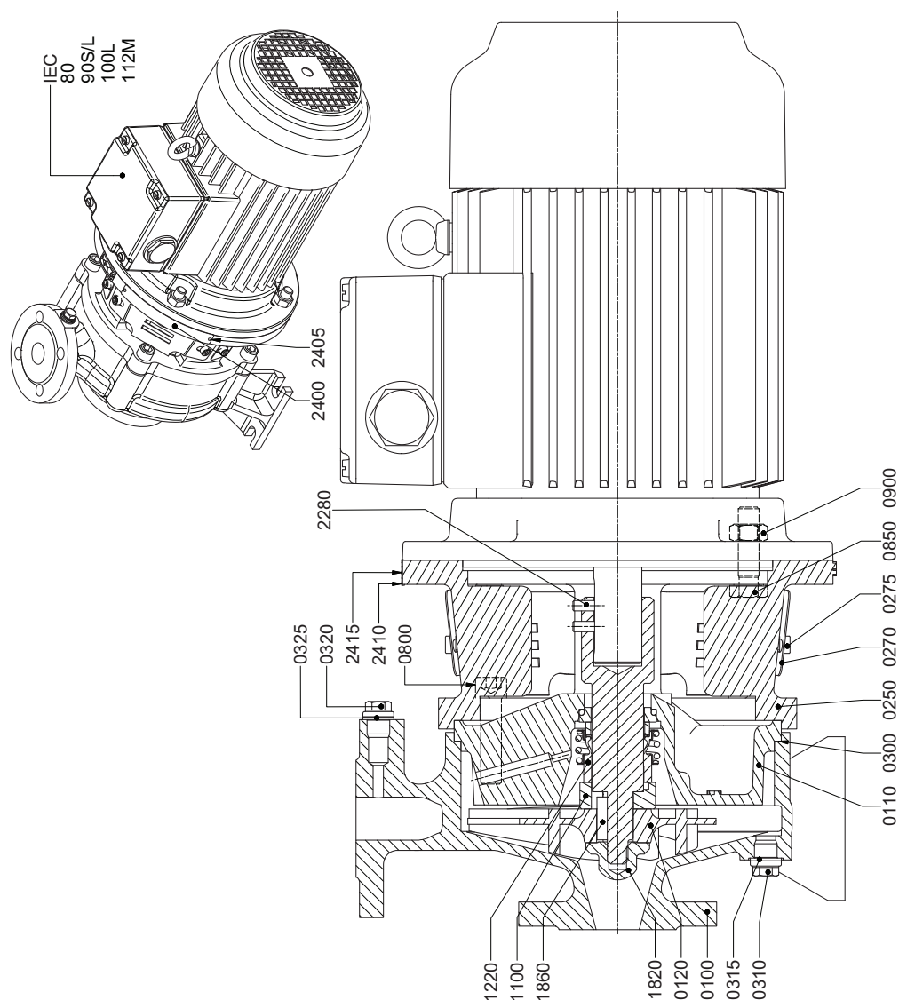
Рисунок 18: Чертеж в разрезе для 25-125, 25-160.
