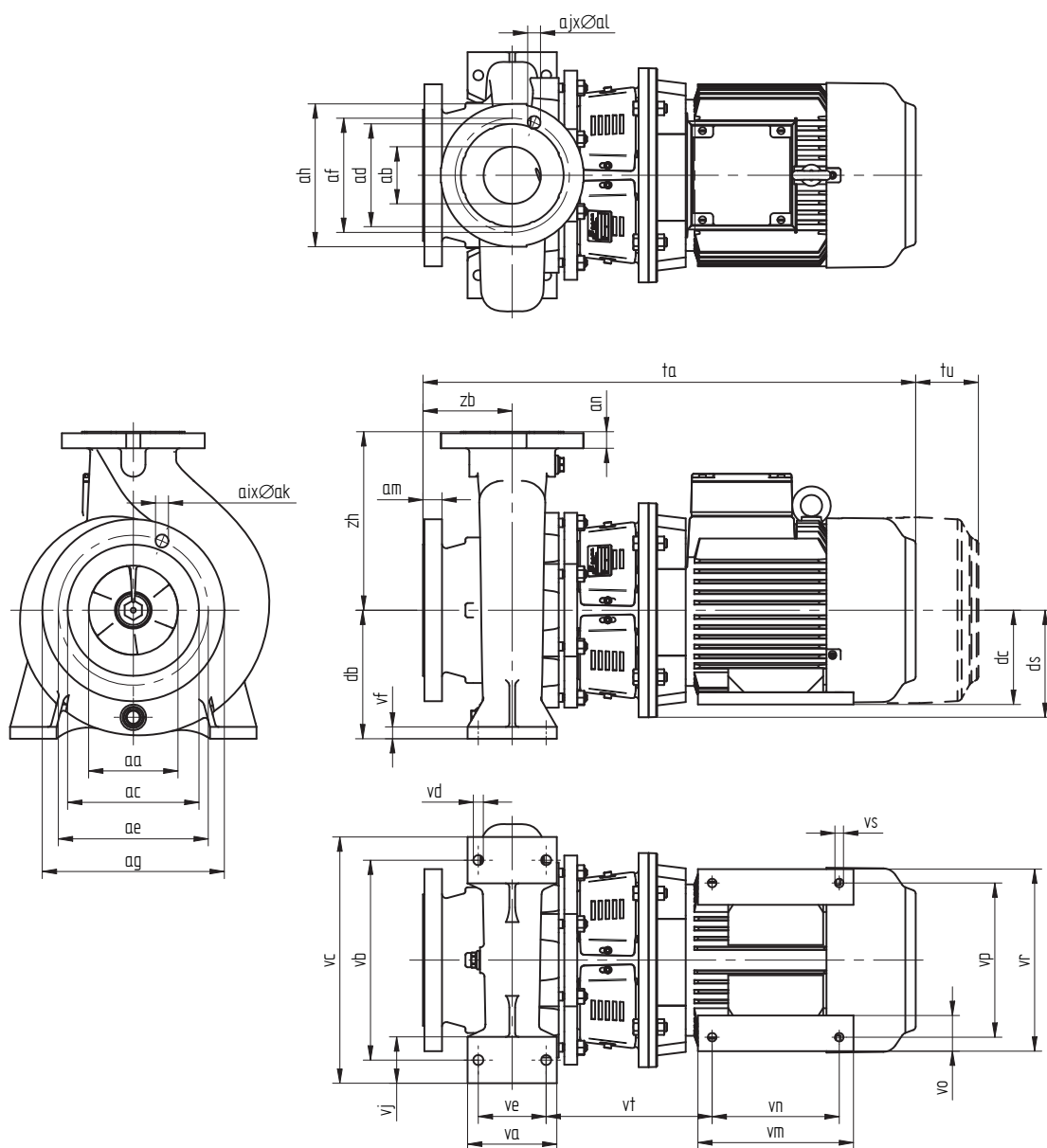
Рисунок 15: Размеры насоса.
