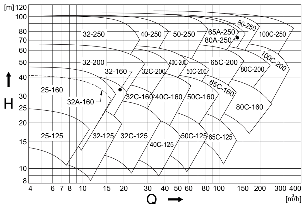
Bild 26: Prestandaöversikt 3000 min -1 .
