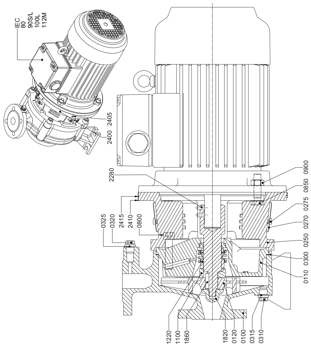
Bild 18: Sektionsritning 25-125, 25-160.
