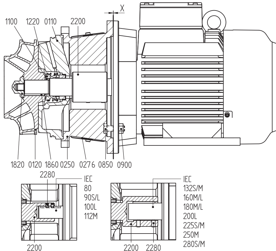
Bild 14: Montering av påsticksaxel
