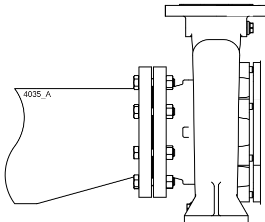
Bild 6: Excentrisk reduktion till inloppsfläns.
