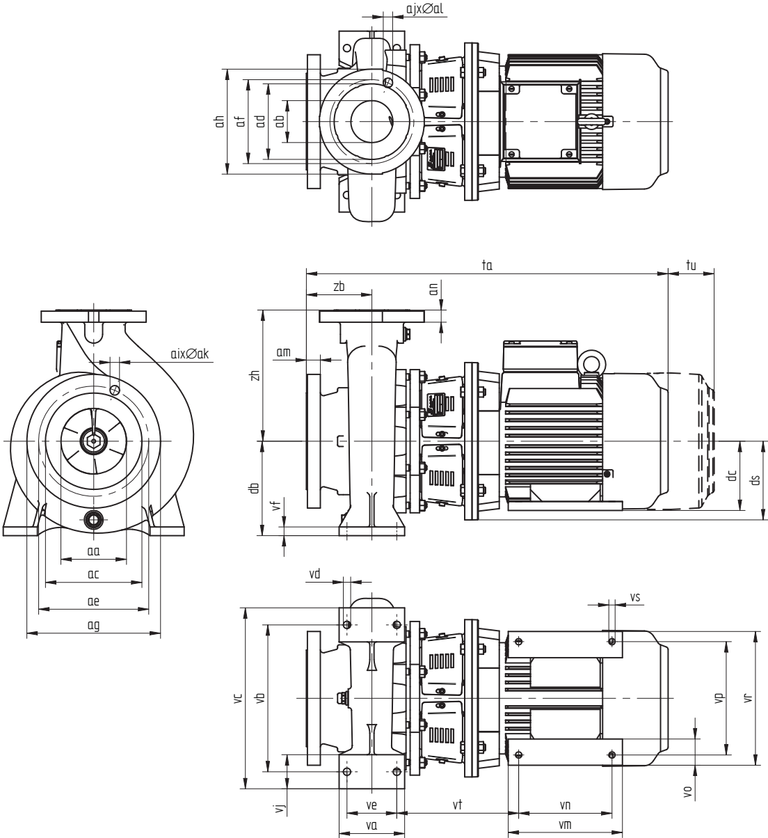
Bild 15: Pumpmått.
