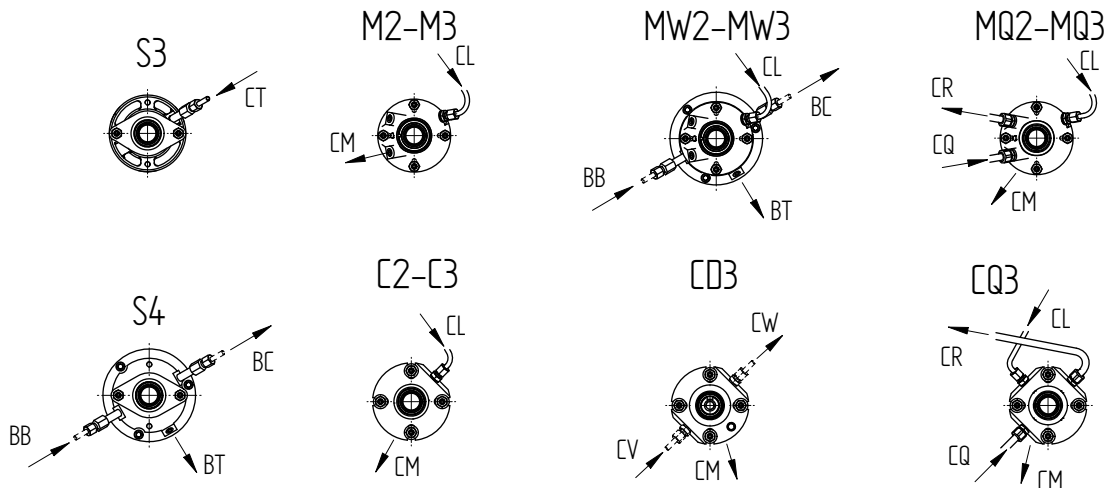
图 35: 轴承组 0、1、2、3 的连接
