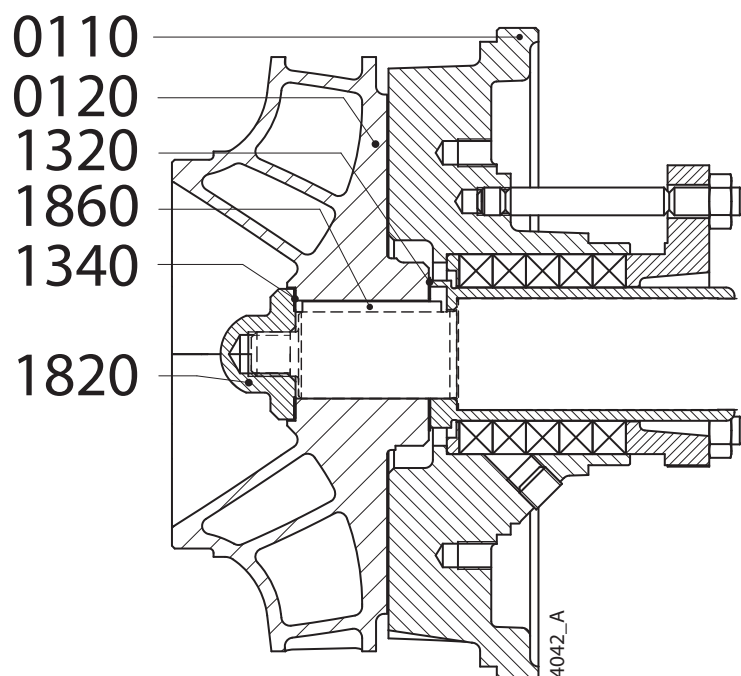
图 18: 拆卸叶轮。
