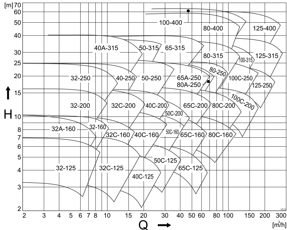
图 90: 性能概述 1500 \text{ min}^{-1} (G、NG、B)。
