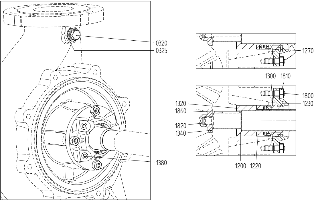
图 58: 机械密封 M7N。
