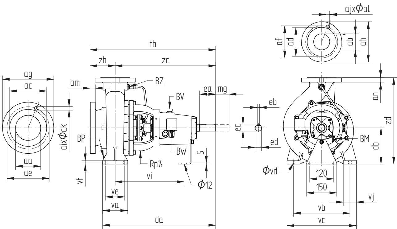
图 36: 泵尺寸 - 周承租 0, 1, 2, 3。
