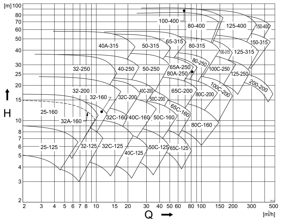
图 96: 性能概述 1800 \text{ min}^{-1} (R)。
