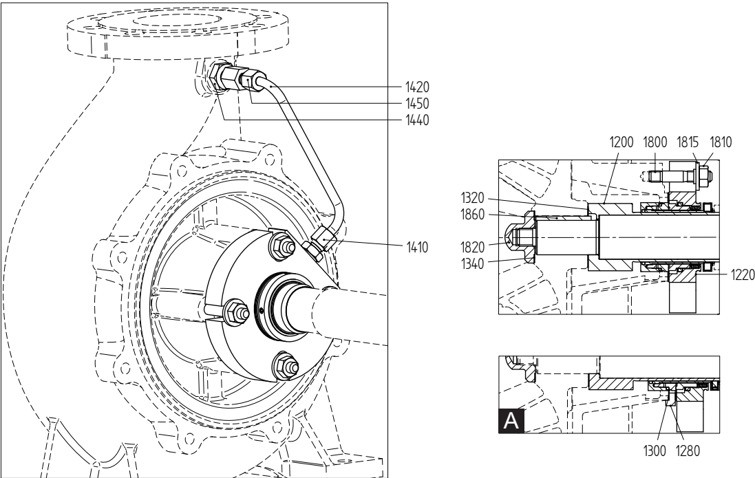
图 82: 机械密封 C3 - CARTEX SN (A = 轴承组 3)。
