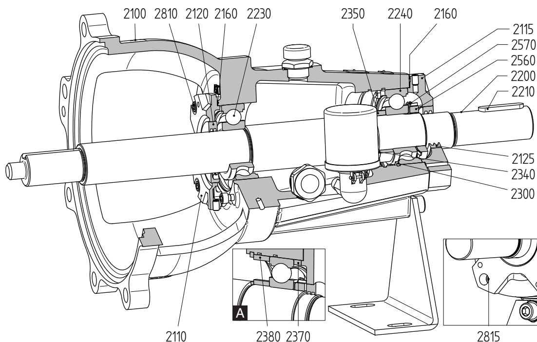
图 28: 轴承 L3（标准，油润滑）（A = 轴承组 3）。
