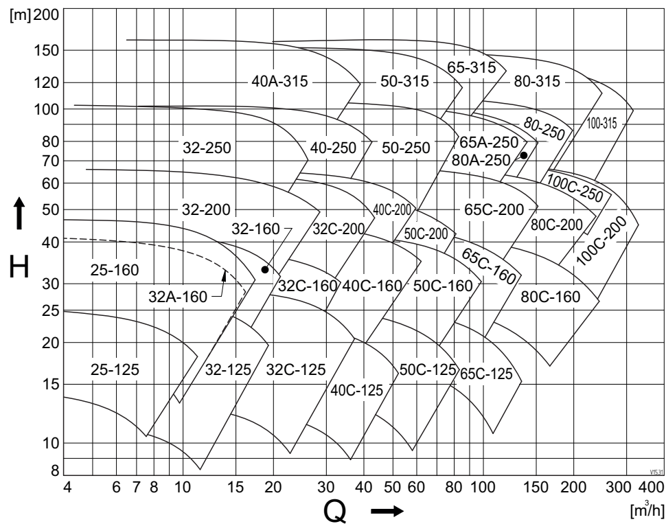
图 93: 性能概述 3000 \text{ min}^{-1} (R)。
