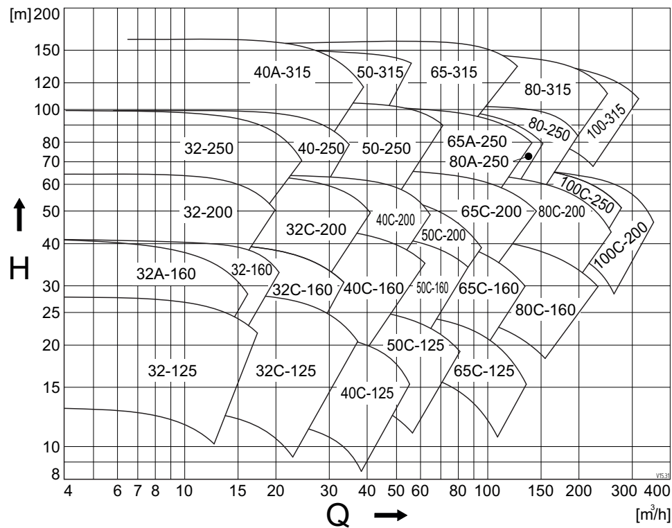
图 89: 性能概述 3000 \text{ min}^{-1} (G、NG、B)。
