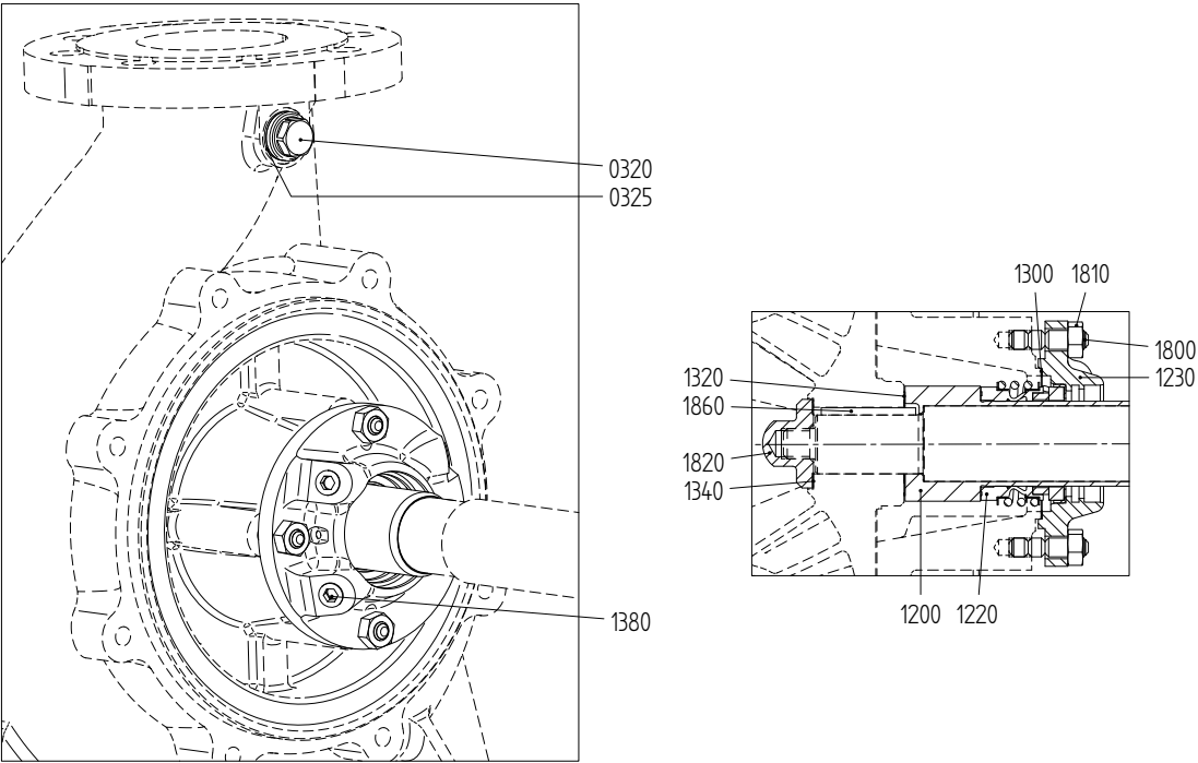
图 59: 机械密封 MG12-G60。
