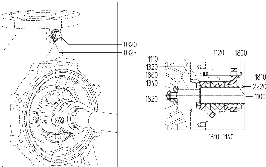
图 53: 填料盒填料 S2。
