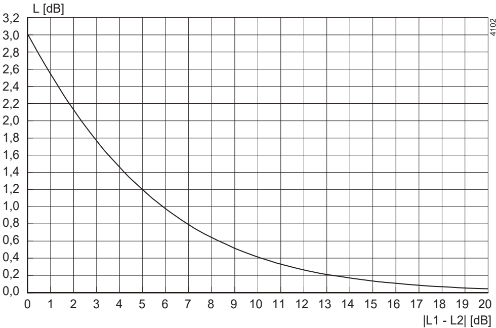
图 99: 整个泵组的噪声级。
