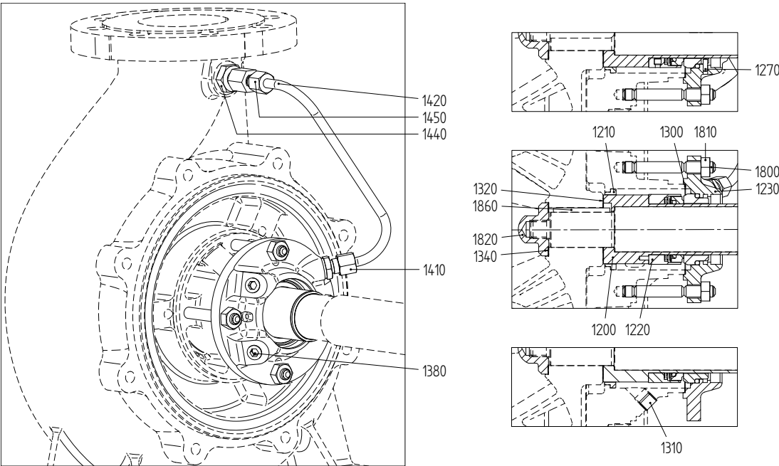
图 56: 机械密封 M7N。
