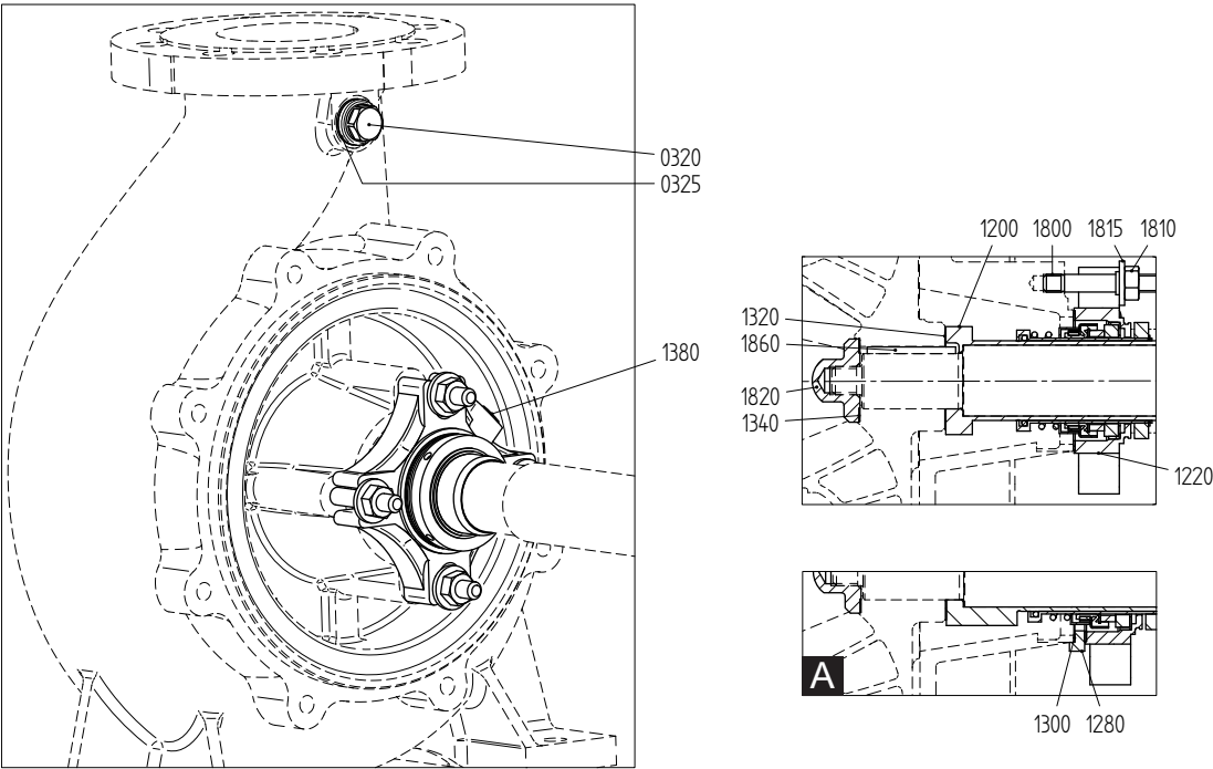
图 78: 机械密封 C2 - UNITEX (A = 轴承组 2 和 3)。
