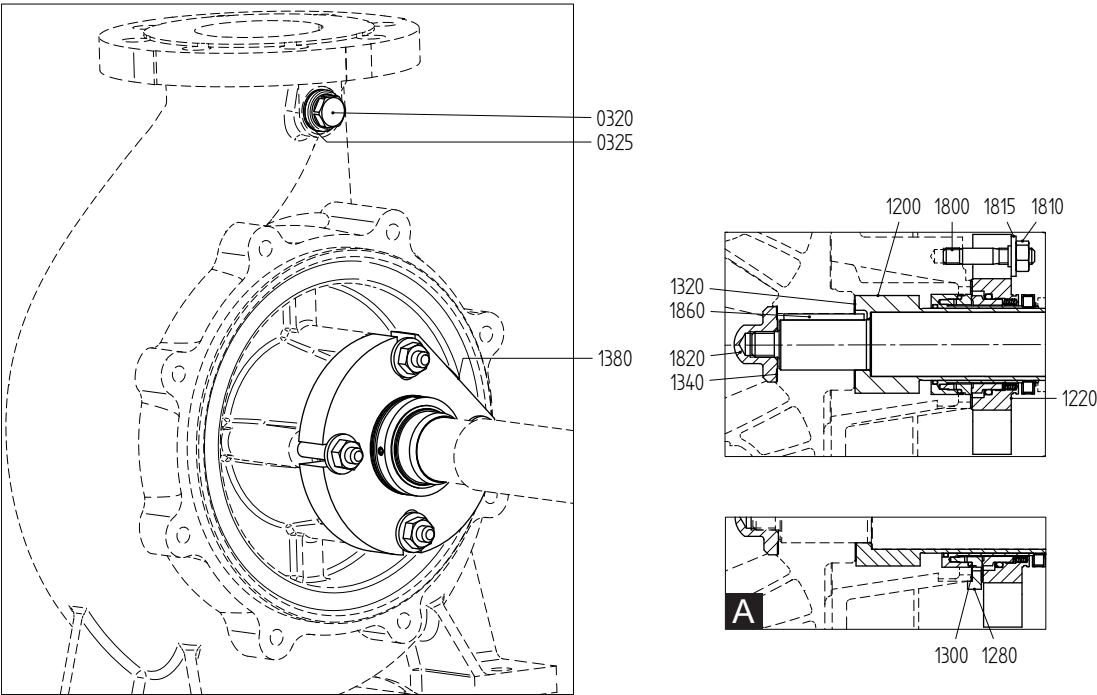
图 81: 机械密封 C3 - CARTEX SN (A = 轴承组 3)。
