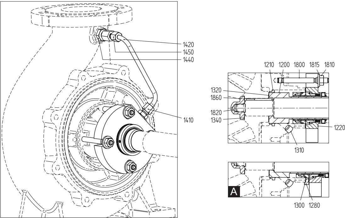
图 80: 机械密封 C3 - CARTEX SN (A = 轴承组 3)。
