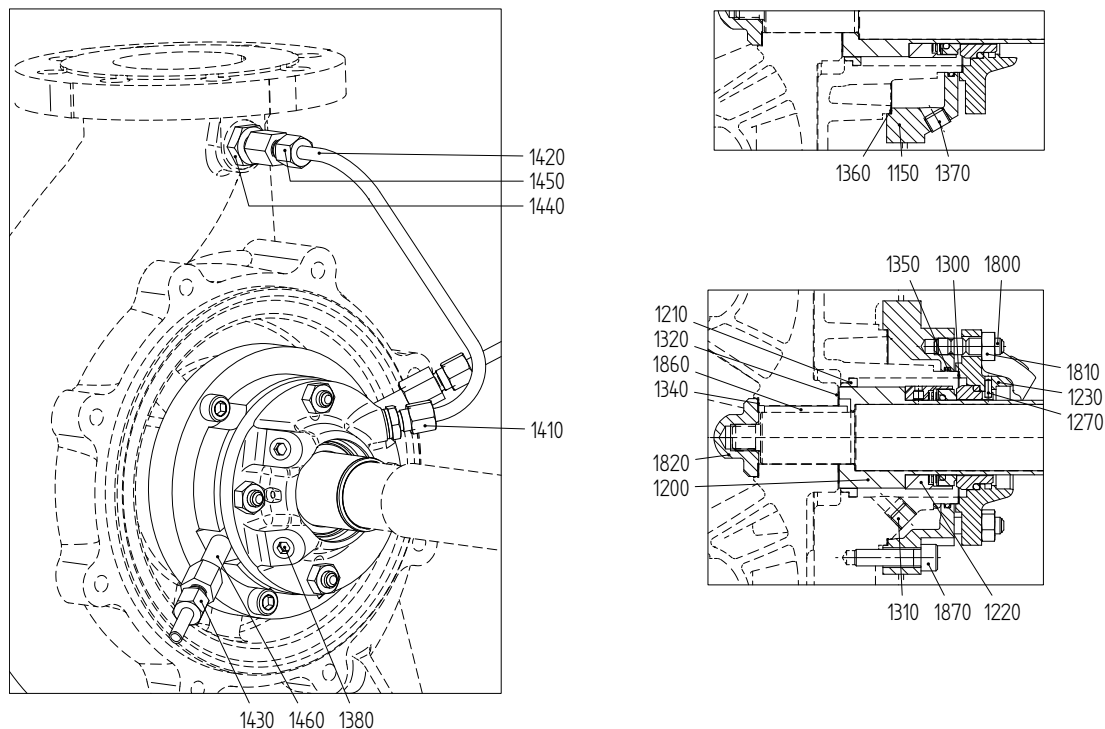
图 25: 机械密封 MW...
