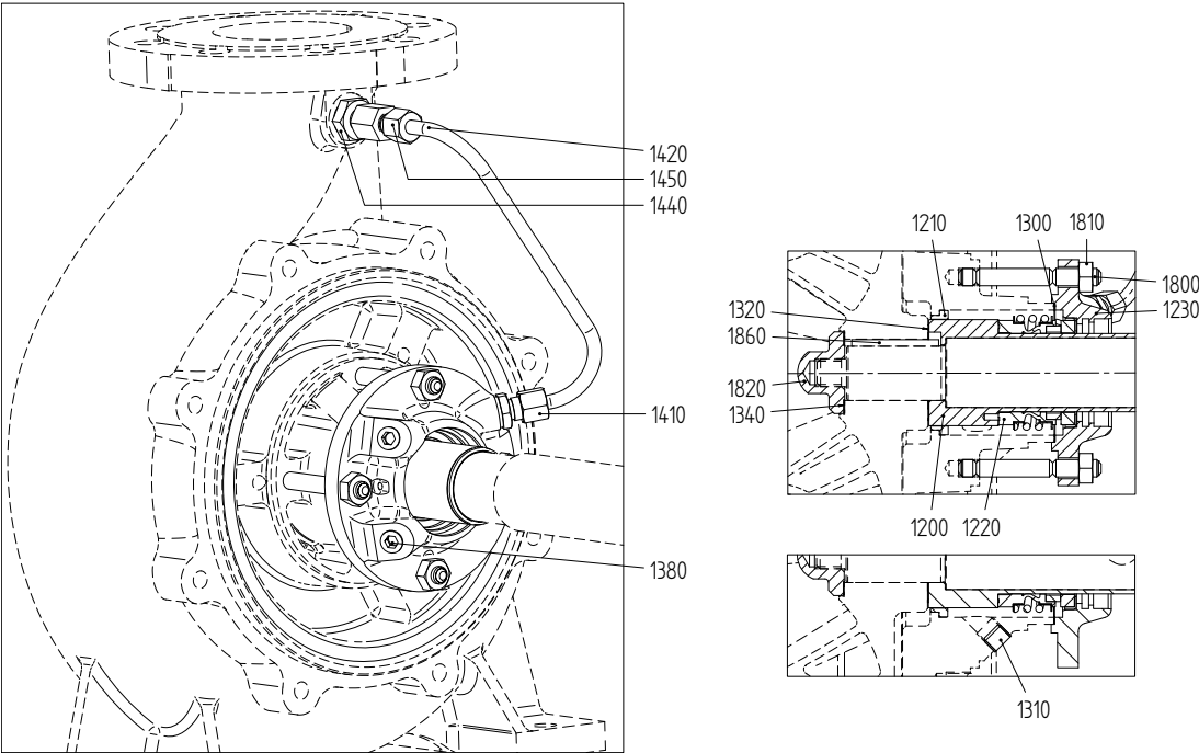
图 57: 机械密封 MG12-G60。
