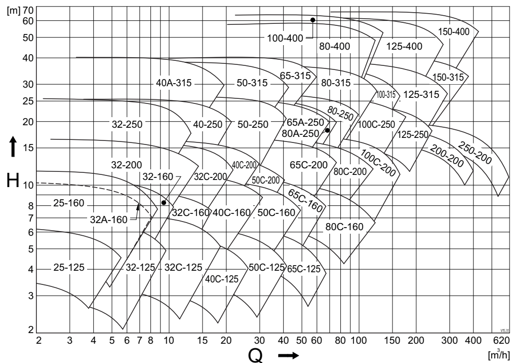
图 94: 性能概述 1500 \text{ min}^{-1} (R)。
