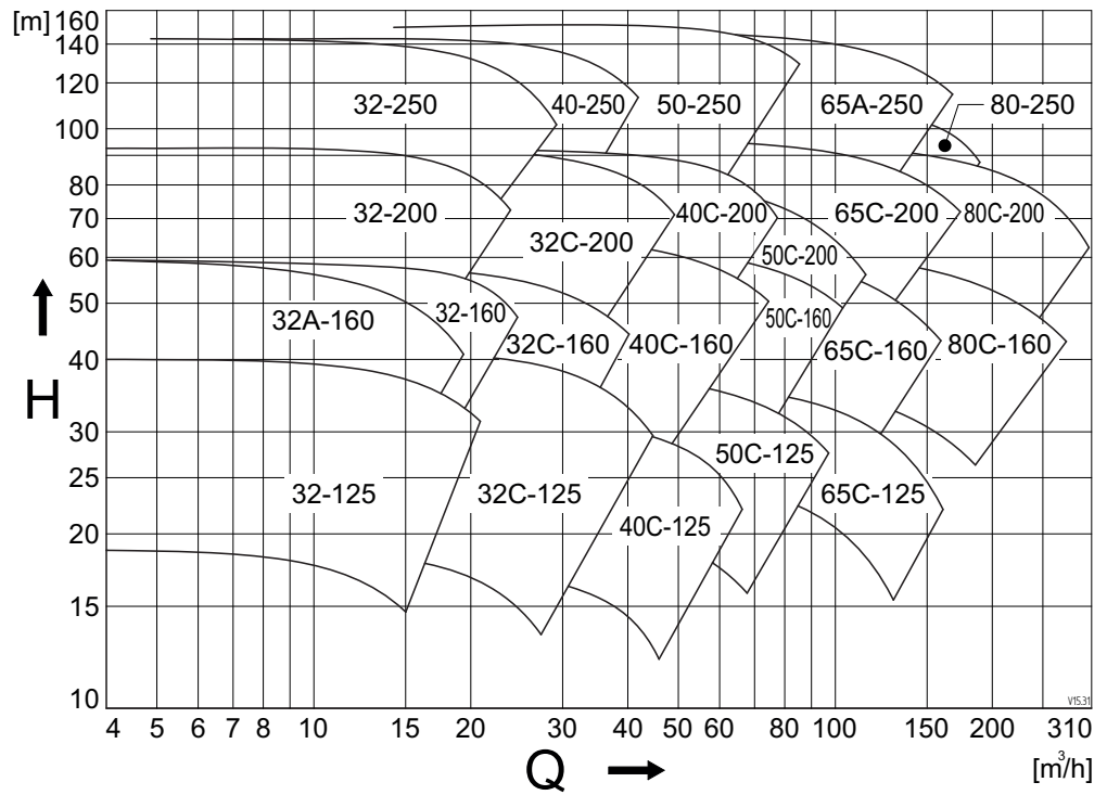
图 91: 性能概述 3600 \text{ min}^{-1} (G、NG、B)。
