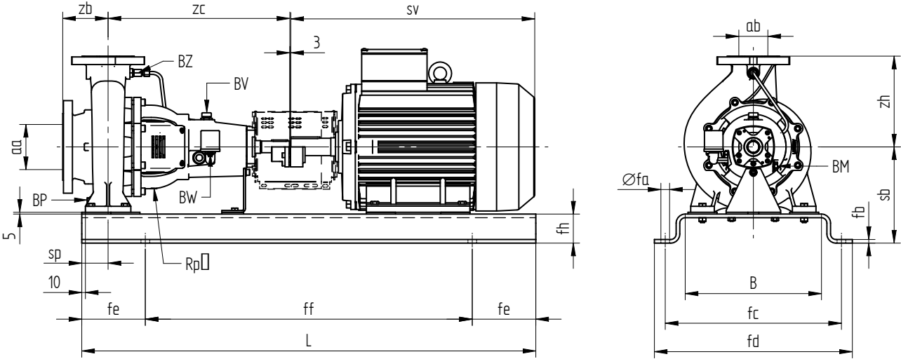
图 37: 泵机组 - 轴承组 0, 1, 2, 3 - 标准联轴器。
