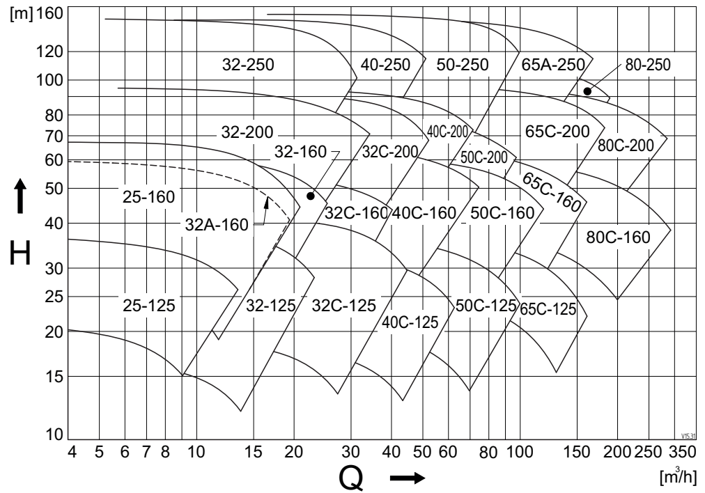
图 95: 性能概述 3600 \text{ min}^{-1} (R)。
