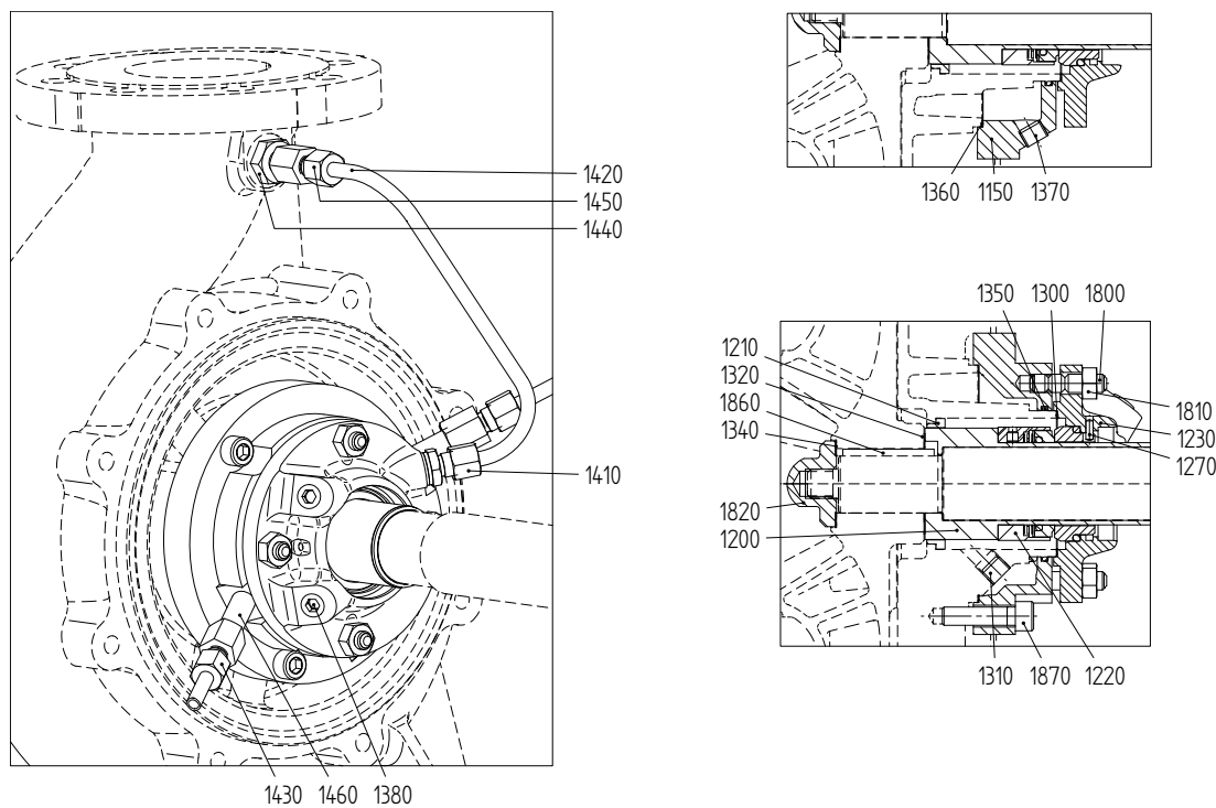
图 74: 机械密封 MW2 - M7N。
