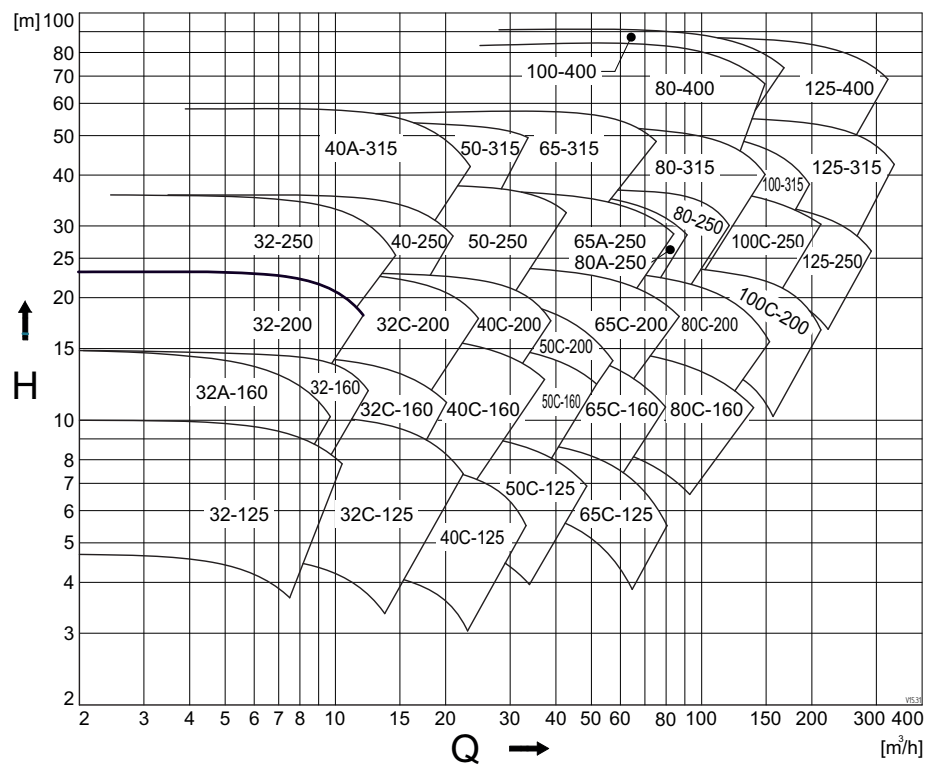
图 92: 性能概述 1800 \text{ min}^{-1} (G、NG、B)。
