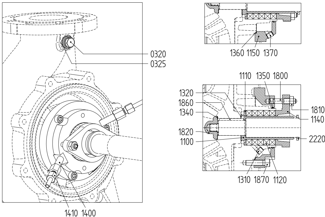
图 55: 填料盒填料 S4。
