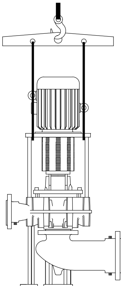
Obrázok 1: Pokyny na zdvíhanie čerpadlovej jednotky.
