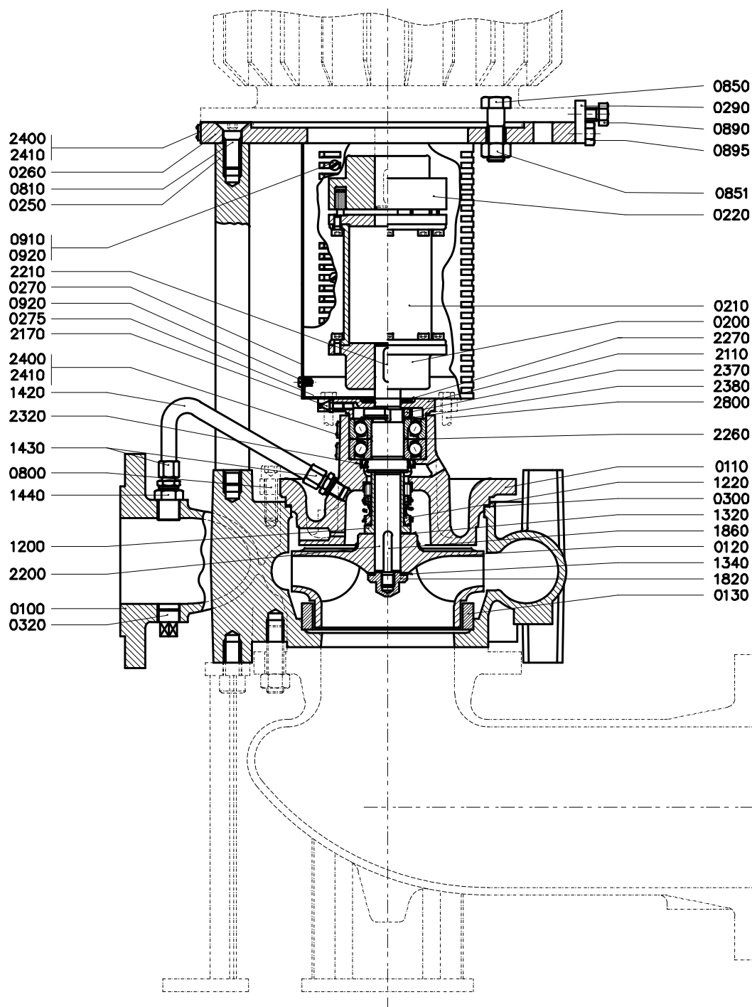
Obrázok 26: Výkres rezu ..-160/..-200/..-250.
