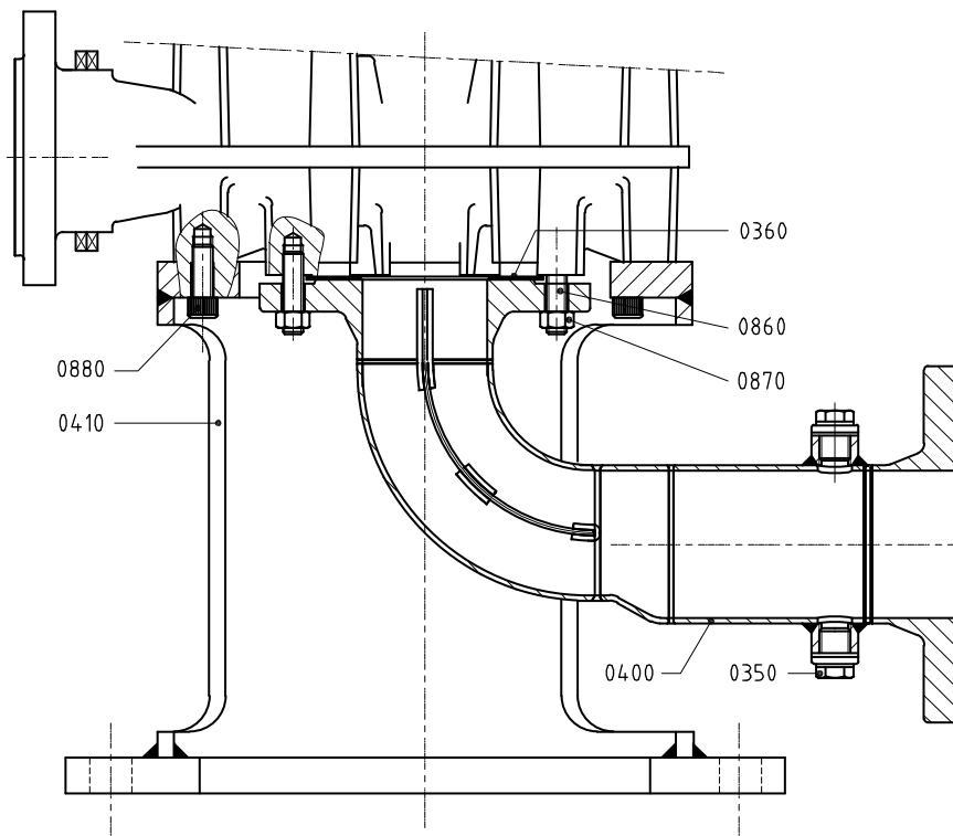
Obrázok 36: Výkres rezu nasávacím ohybom 200-200/250B-315.
