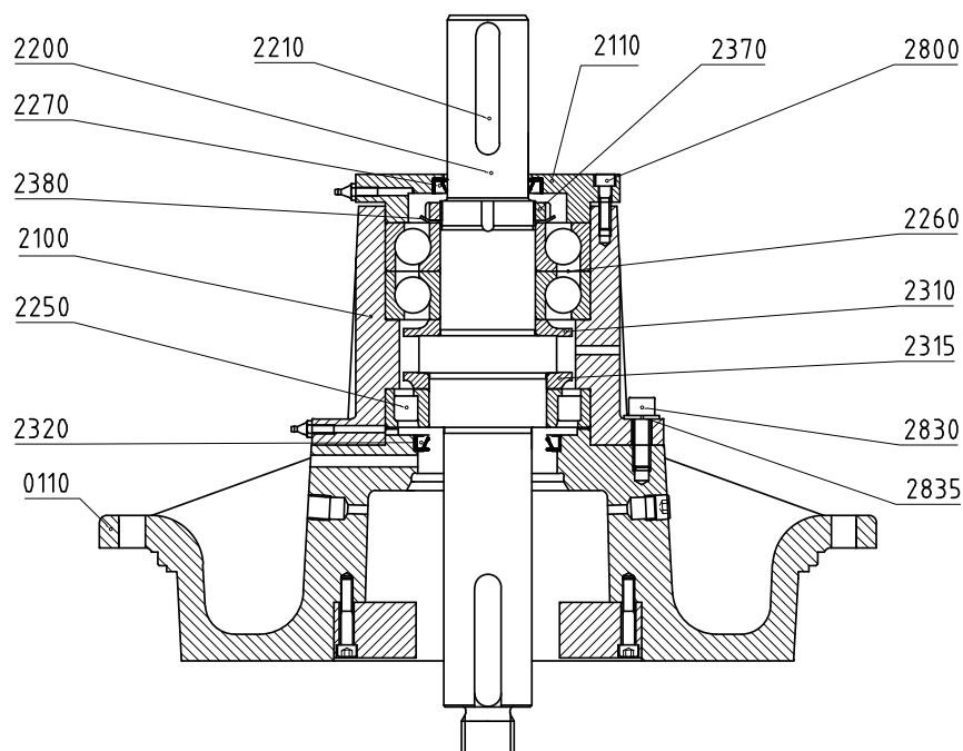
Obrázok 11: Demontáž ložísk 200-400, 250-250, 250-315, 300-250, 300-315.
