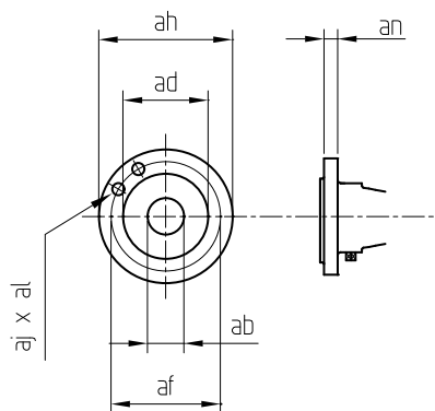
Obrázok 14: Rozmery prívodnej príruby.
