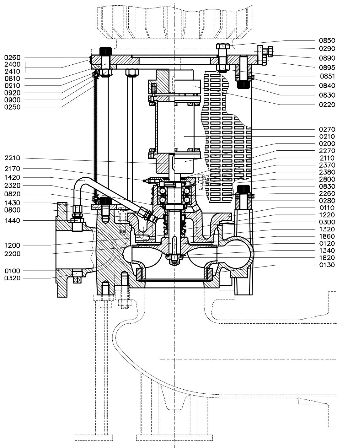
Obrázok 27: Výkres rezu ...-315/...-400.
