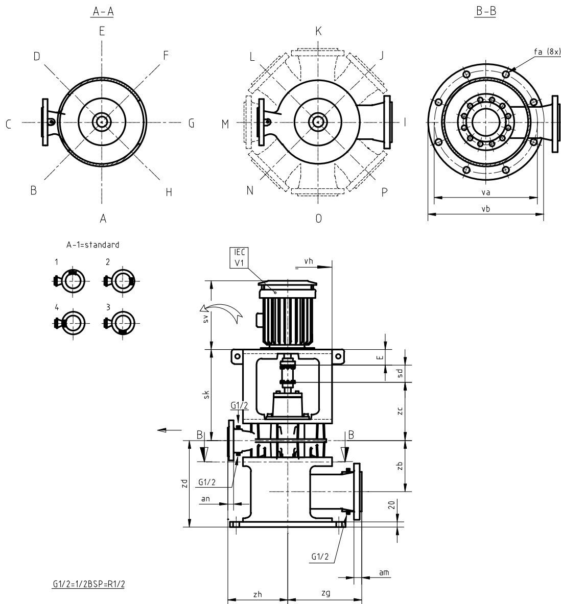
Obrázok 24: Rozměry čerpadla K3, s nasávacím ohybom.
