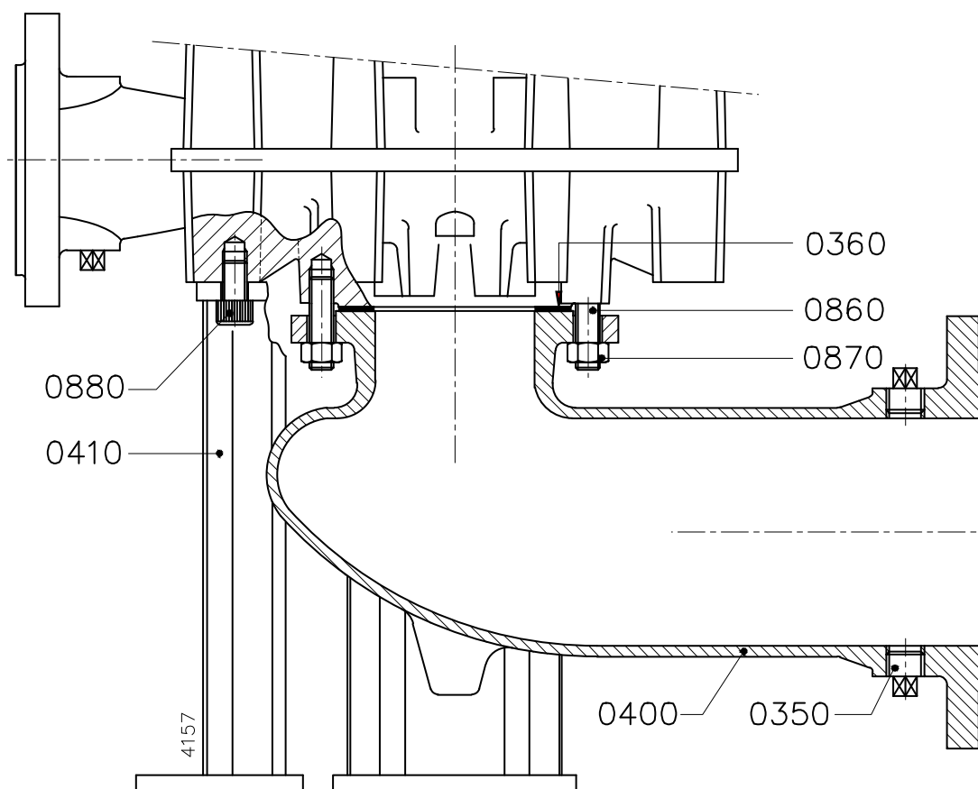
Obrázok 35: Výkres rezu nasávacím ohybom.
