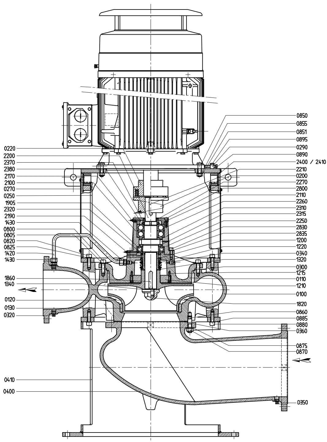
Obrázok 32: Výkres rezu 200-400, 250-250, 250-315, 300-250, 300-315.
