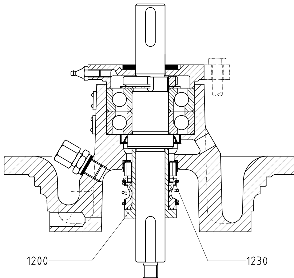
Obrázok 9: Demontáž mechanického tesnenia.
