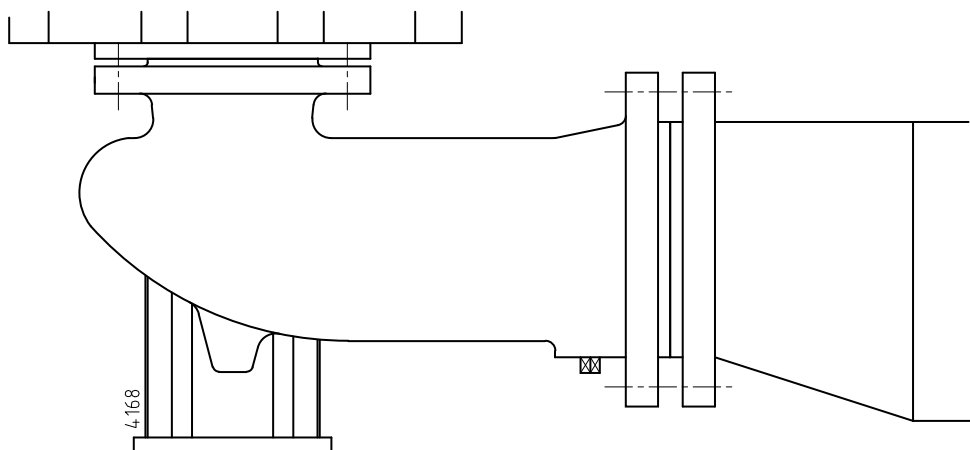
Obrázok 6: Excentrický redukčný ventil k saciej prírubе.
