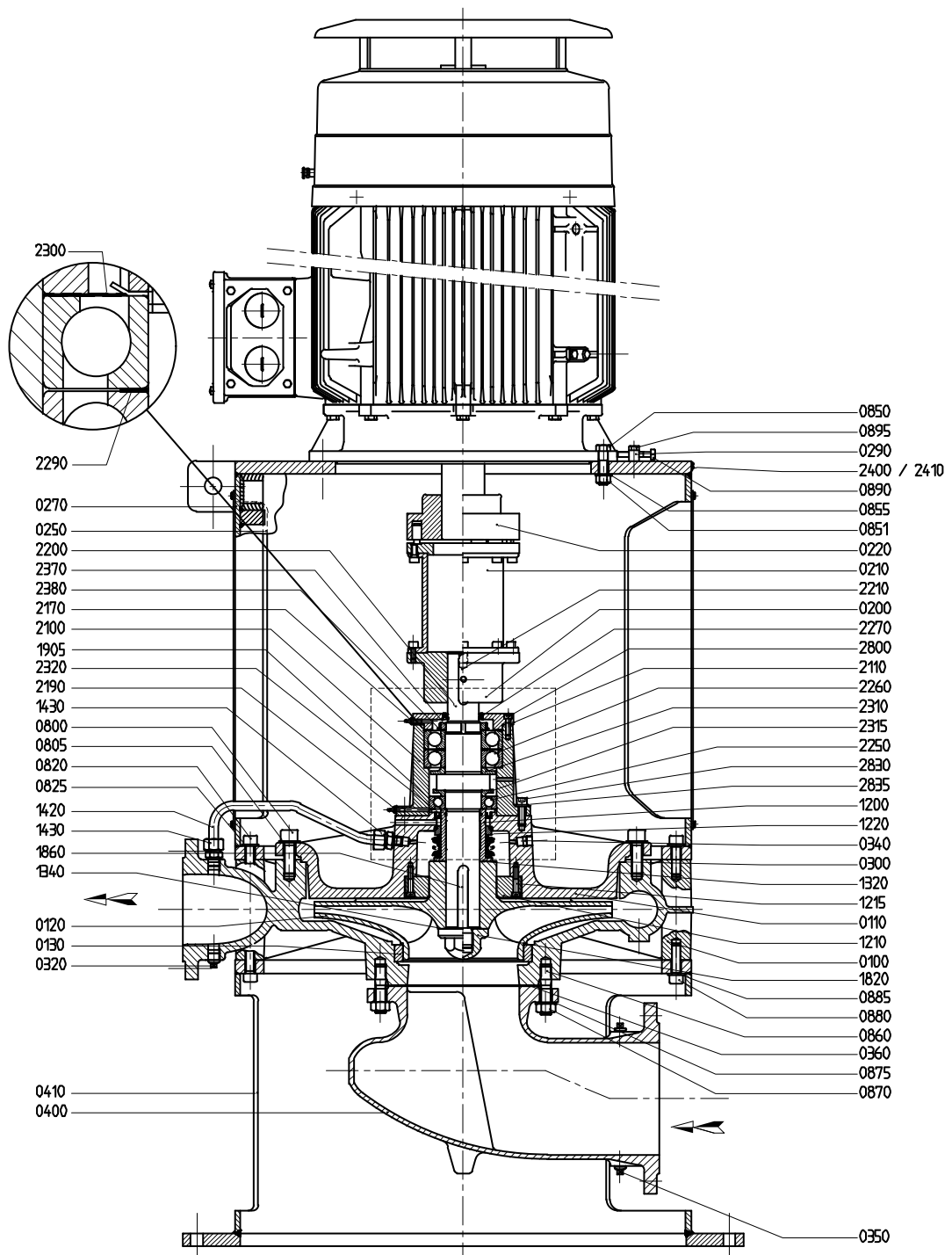
Obrázok 31: Výkres rezu 125-500.
