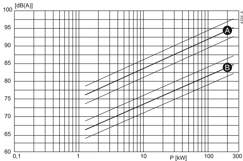
Obrázok 42: Hladina hluku v závislosti od výkonu čerpadla [kW] pri otáčkach 2900 min. -1 A = hladina akustického výkonu, B = hladina akustického tlaku.
