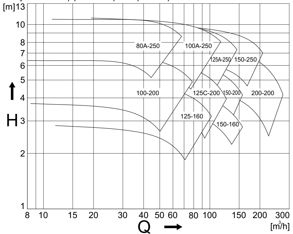
Рисунок 17: Обзор рабочих параметров CL при 950 мин -1 .
