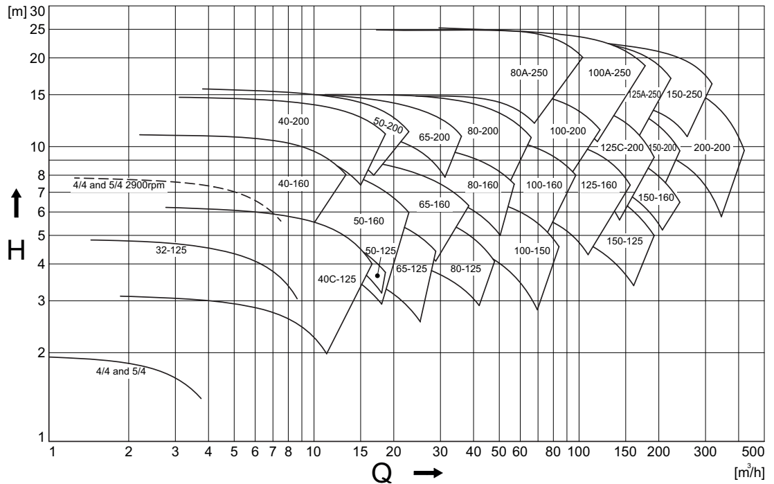
Рисунок 16: Обзор рабочих параметров CL при 1450 мин -1 .
