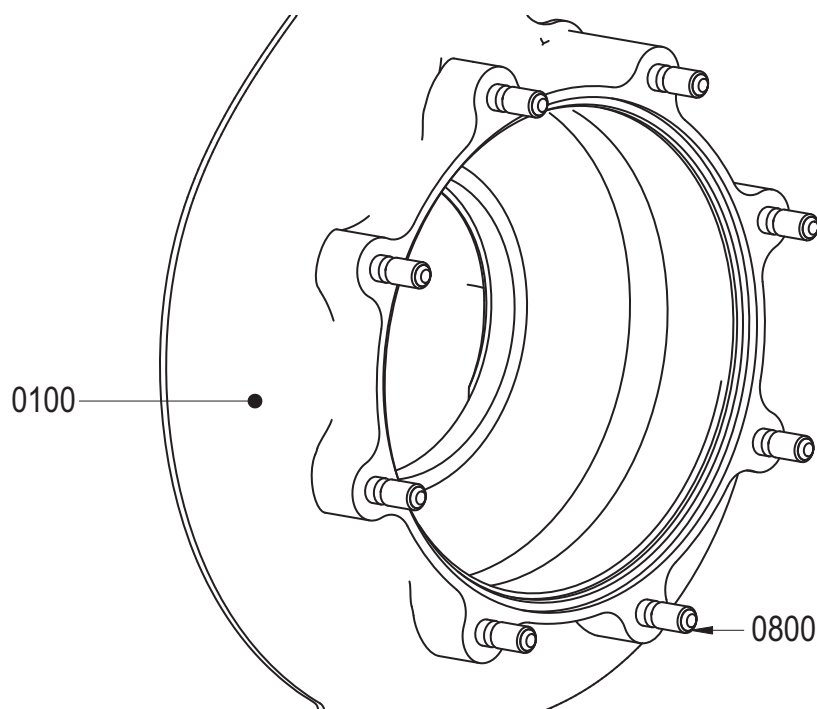
Рисунок 8: Корпус насоса со шпильками.
