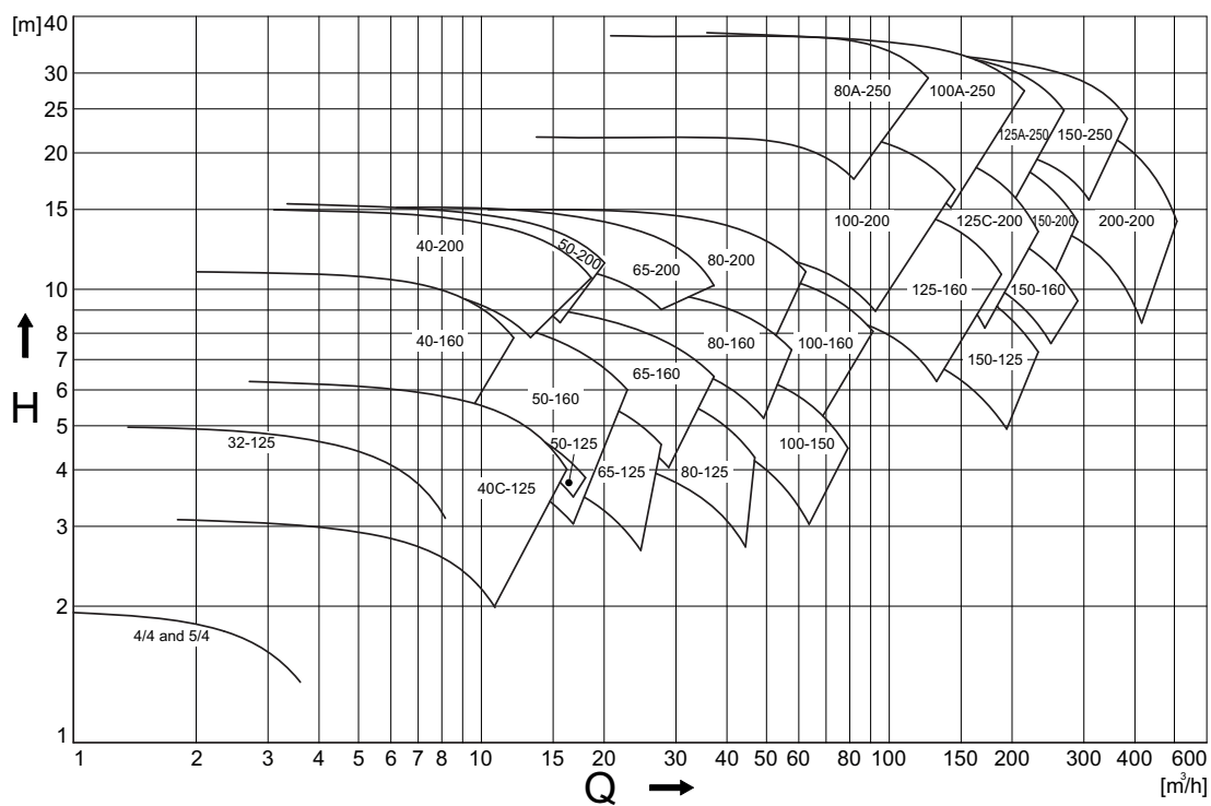
Рисунок 18: Обзор рабочих параметров CL при 1750 мин -1 .
