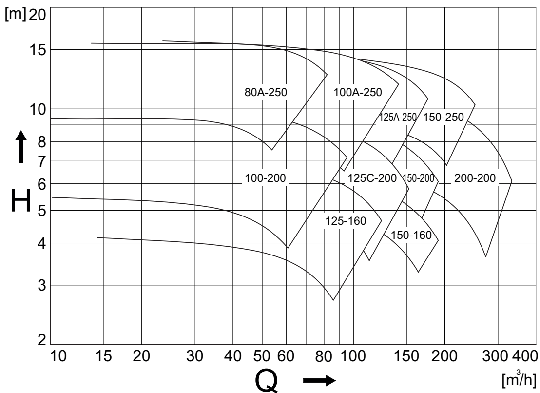
Рисунок 18: Обзор рабочих параметров CL при 1750 мин -1 .
