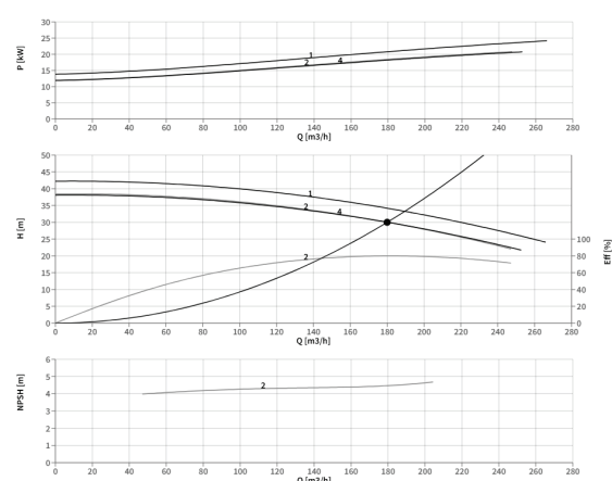
Рисунок 2: Hydraulic Investigator 3 (HI-3)
