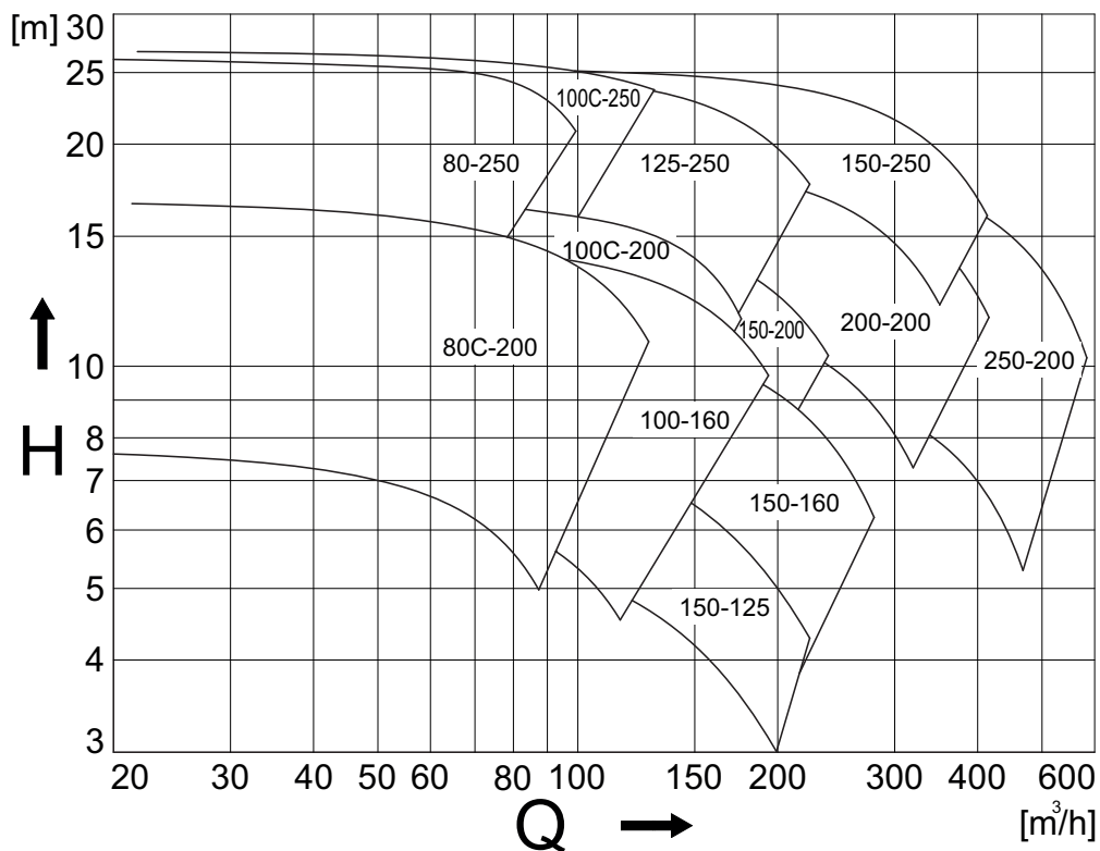
Рисунок 20: Обзор рабочих параметров СВН при 1450 мин -1 .
