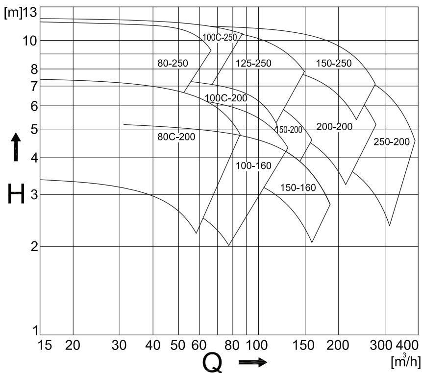
Рисунок 21: Обзор рабочих параметров СВН при 950 мин -1 .
