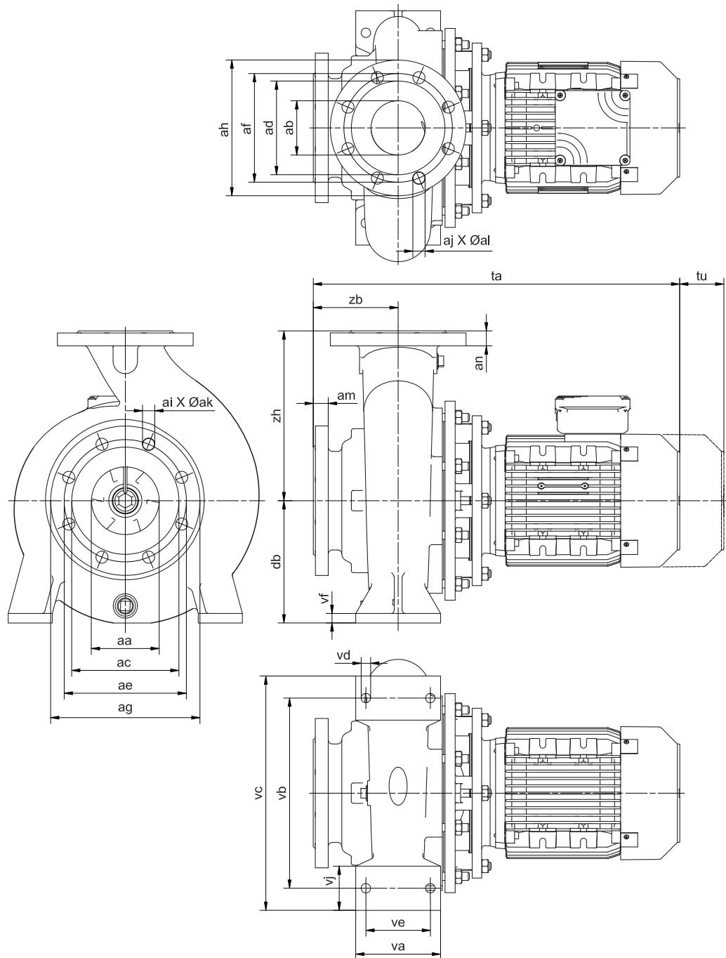
Рисунок 12: Размеры насоса CombiBlocHorti.
