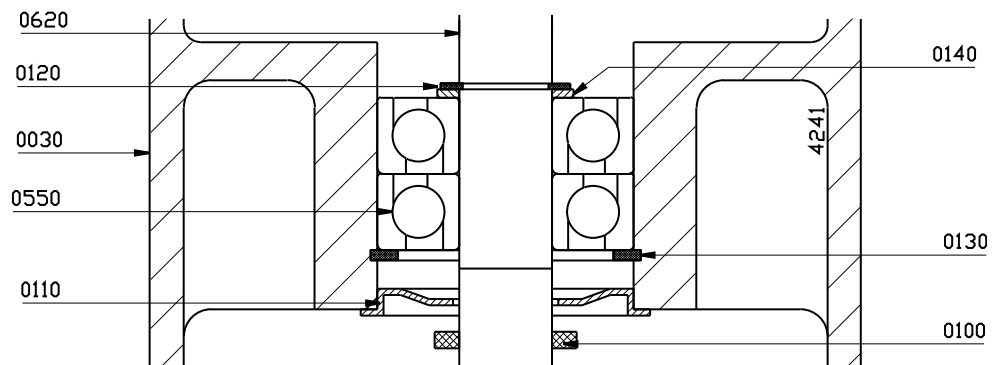
Kuva 8: Kuulalaakereiden asennus.
