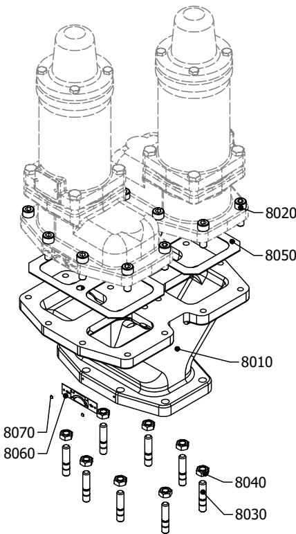
Dubbel säkerhetsventil – vertikal
