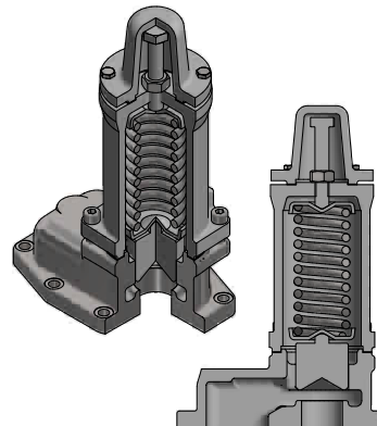
Säkerhetsventil – vertikal
