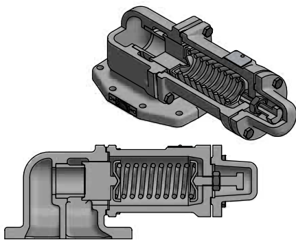
Säkerhetsventil – horisontell
