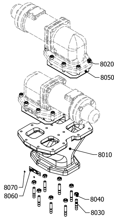
Dubbel säkerhetsventil – horisontell
