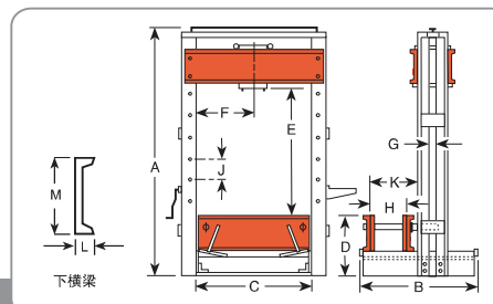
外形尺寸
