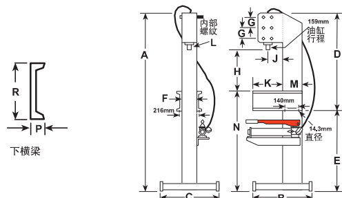
外形尺寸
