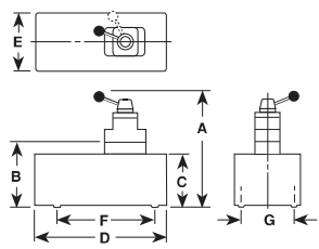
典型配置 适用于连接单作用油缸
