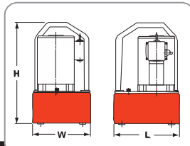
外形尺寸 (mm)
