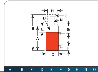
30, 60, 100吨双作用 油缸，颈部带安装螺纹
