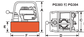
PG303 和 PG304
