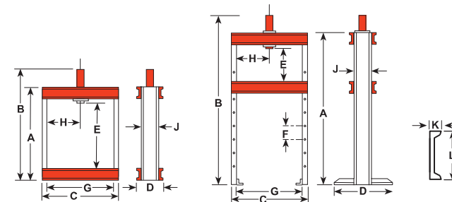
外形尺寸
