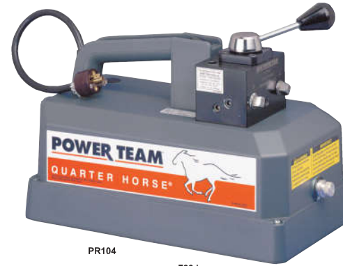
Quarter Horse液压泵最大操作力为700bar，能涵盖大多数的手动液压工具。
